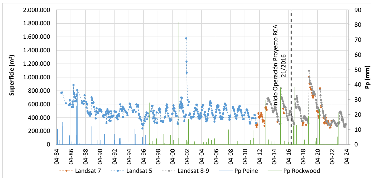
Figura N°6-9. Variación histórica Sistema Lagunar Peine, Landsat NDWI (1985-2024)
