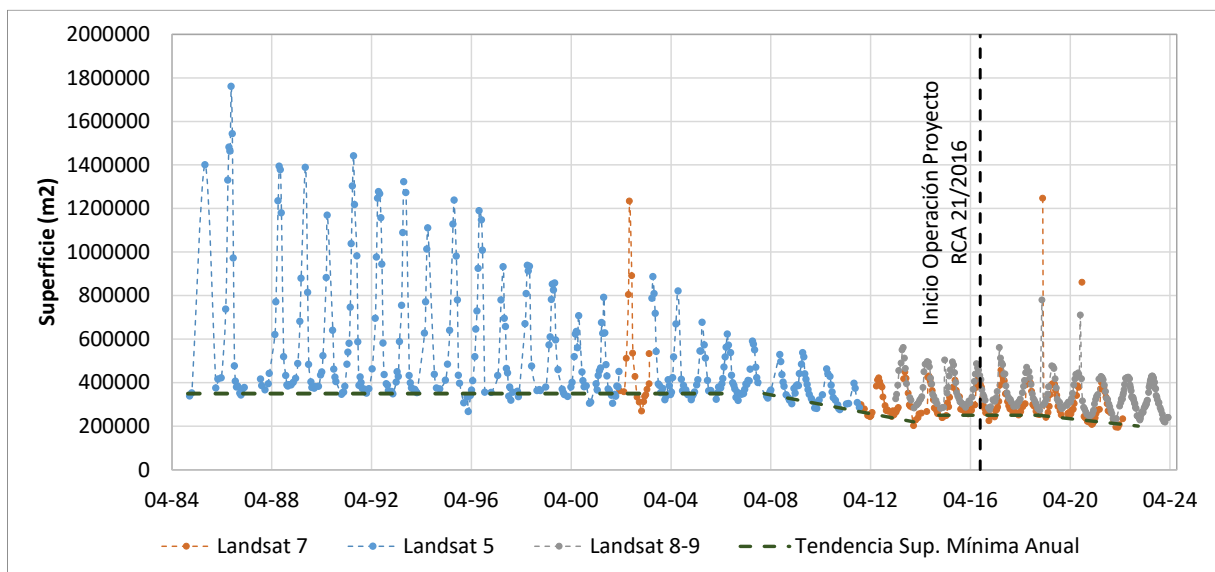
Figura N°6-4. Variación histórica Sistema Lagunar La Punta-La Brava, Landsat NDWI (1985-2024).
