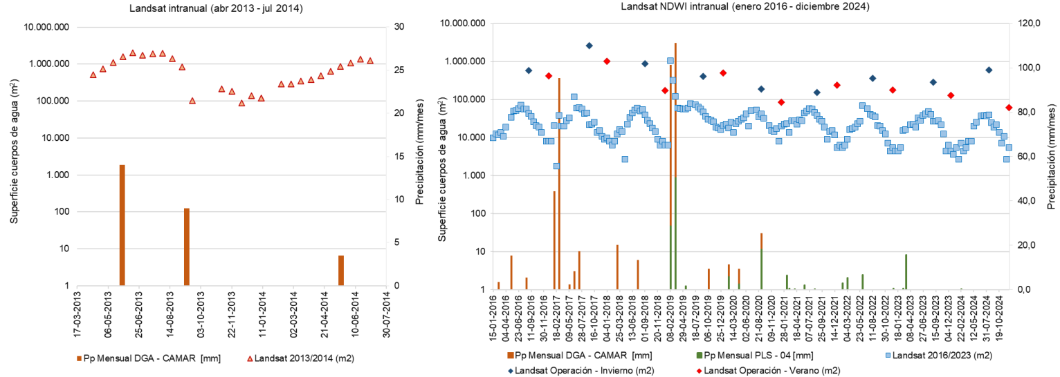
Figura N°6-13. Variación intranual de las superficies lagunares mediante el uso de imágenes Landsat, Sector Aguas de Quelana.
