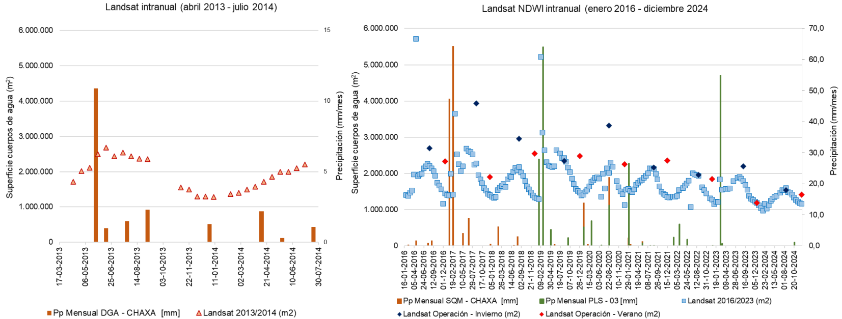
Figura N°6-17. Variación intranual de las superficies lagunares mediante el uso de imágenes Landsat, Sector Soncor.
